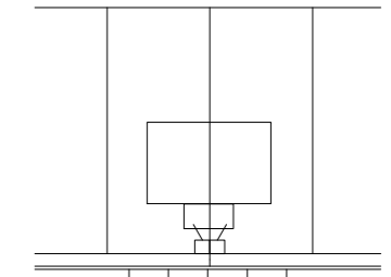
DETALLE INSTALACIÓN Y CONEXIÓN EQUIPO DE MEDIDA B.T. < 15 KV
